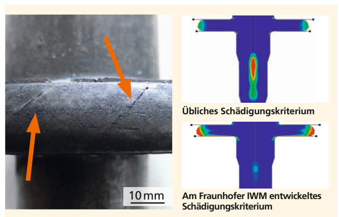
2 Verbesserung der Schadensvorhersage am Beispiel einer Getriebewelle: Das neu entwickelte Materialmodell sagt die tatsächlichen Schadensorte am Bauteil genauer voraus.
