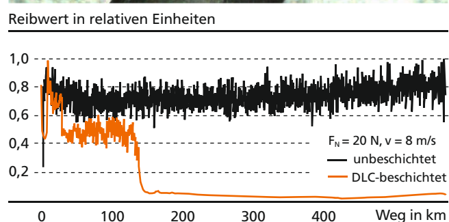
1 DLC-beschichtete Elastomerdichtung (oben), Vergleich der Reibwerte eines beschichteten und unbeschichteten Elastomers (unten).
