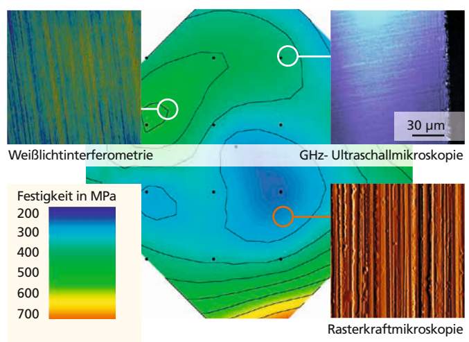
1 Ermittelte Festigkeitsverteilung eines Si-Wafers nach dem Abdünnen in Kombination zur Bewertung der Oberflächenbeschaffenheit.
