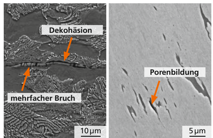
1 Beobachtete Mechanismen zur Porenbildung an typischerweise vorzufindenden Mangansulfid-Teilchen: Dekohäsion und Bruch (links), Abscheren durch Druckumformung (rechts).
